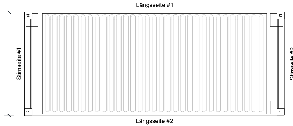
Draufsicht Dach
